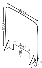
Kleines Modell - Thekenaufsatz
