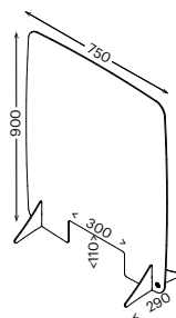
Erhöhtes Modell - Thekenaufsatz
