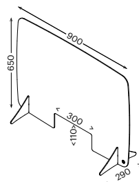
Großes Modell - Thekenaufsatz
